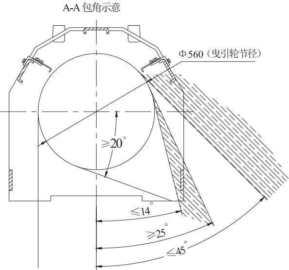
注：钢丝绳绕出角度按上图所示范围，避开阴影部分
