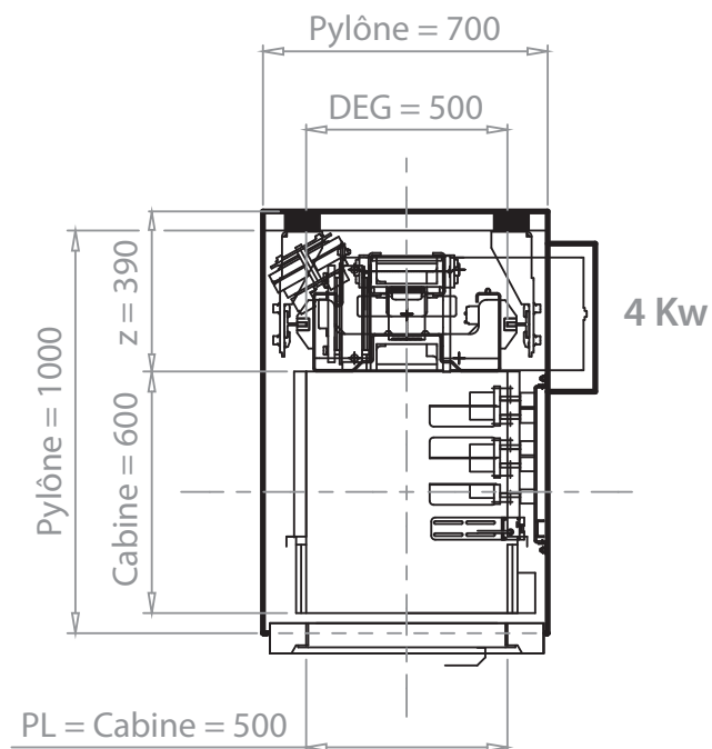
180 kg - DEG 500 - Simple accès
