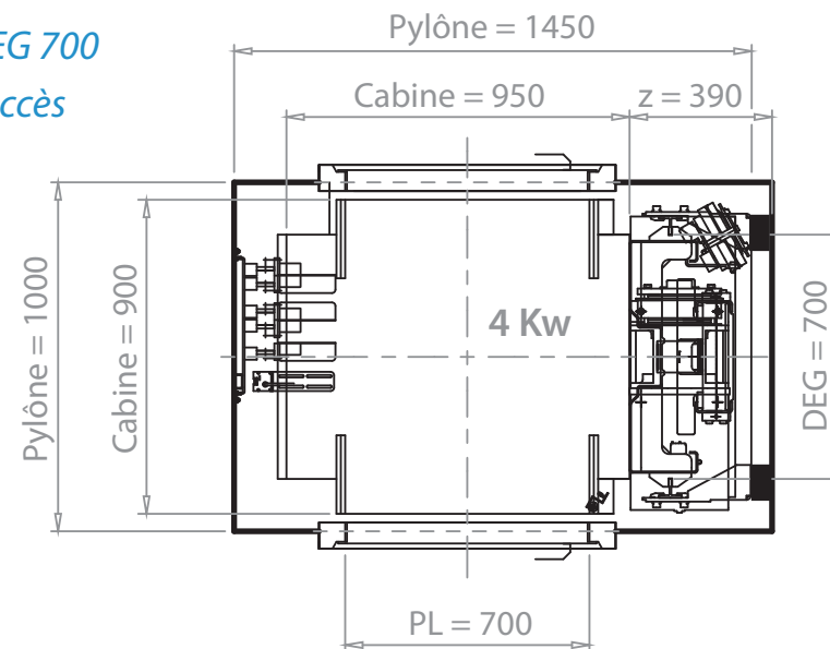
450 kg - DEG 900 Accès d'équerre
